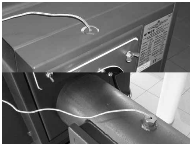
Rys. 14 – Widok czujnika temperatury spalin TS lub TSV podłączonego do łącznika kominowego. Przypadku kotłów D30P, D31P, D40P i D50P znajduje się na kanale dymowym kotła.
